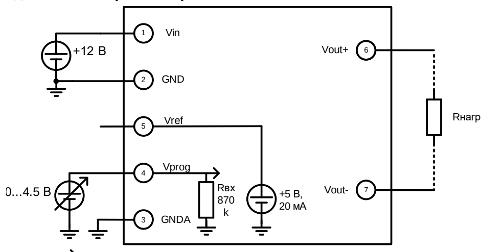
Рис.2 – Схема подключения
