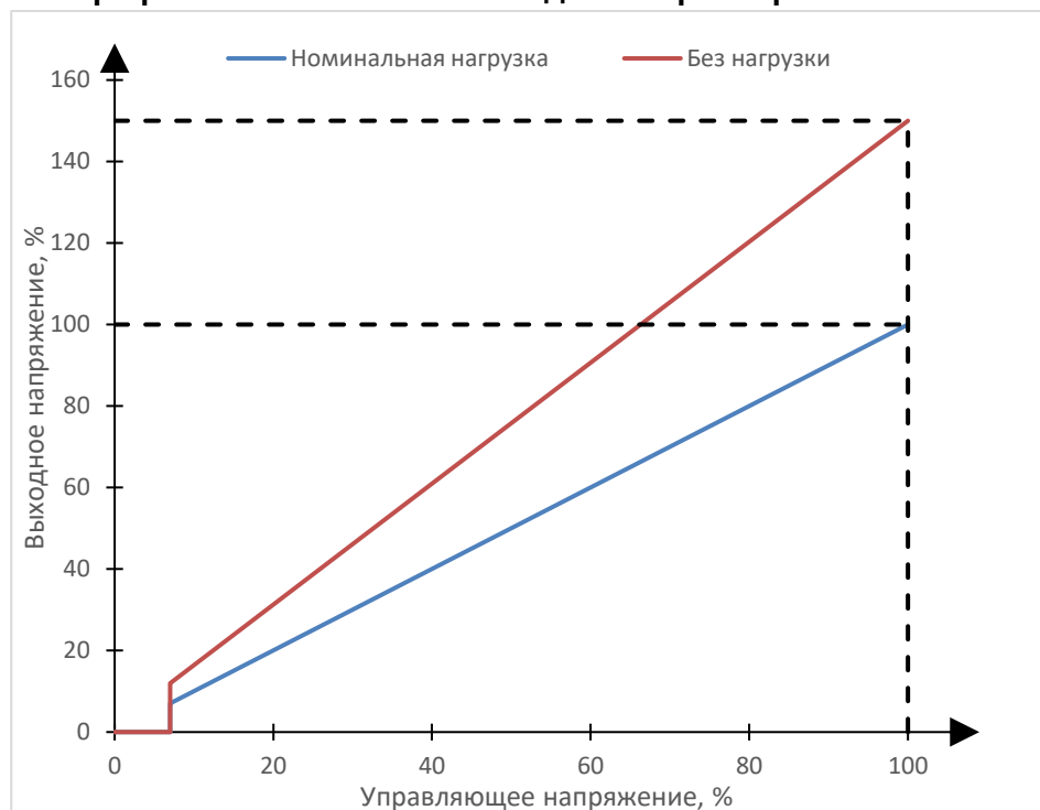
Рис. 3 – График зависимости выходного напряжения от нагрузки
