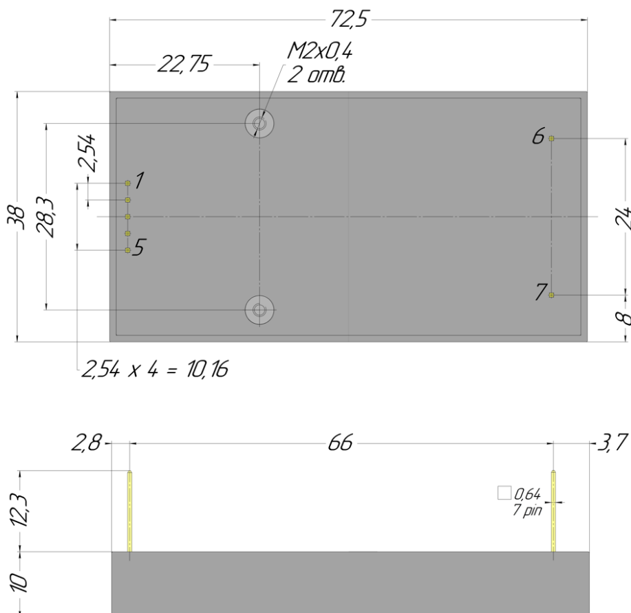
Рис.5 – Общий вид источника
