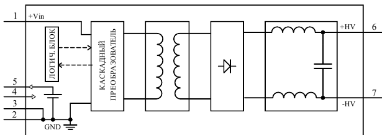
Рис. 1 – Функциональная схема
